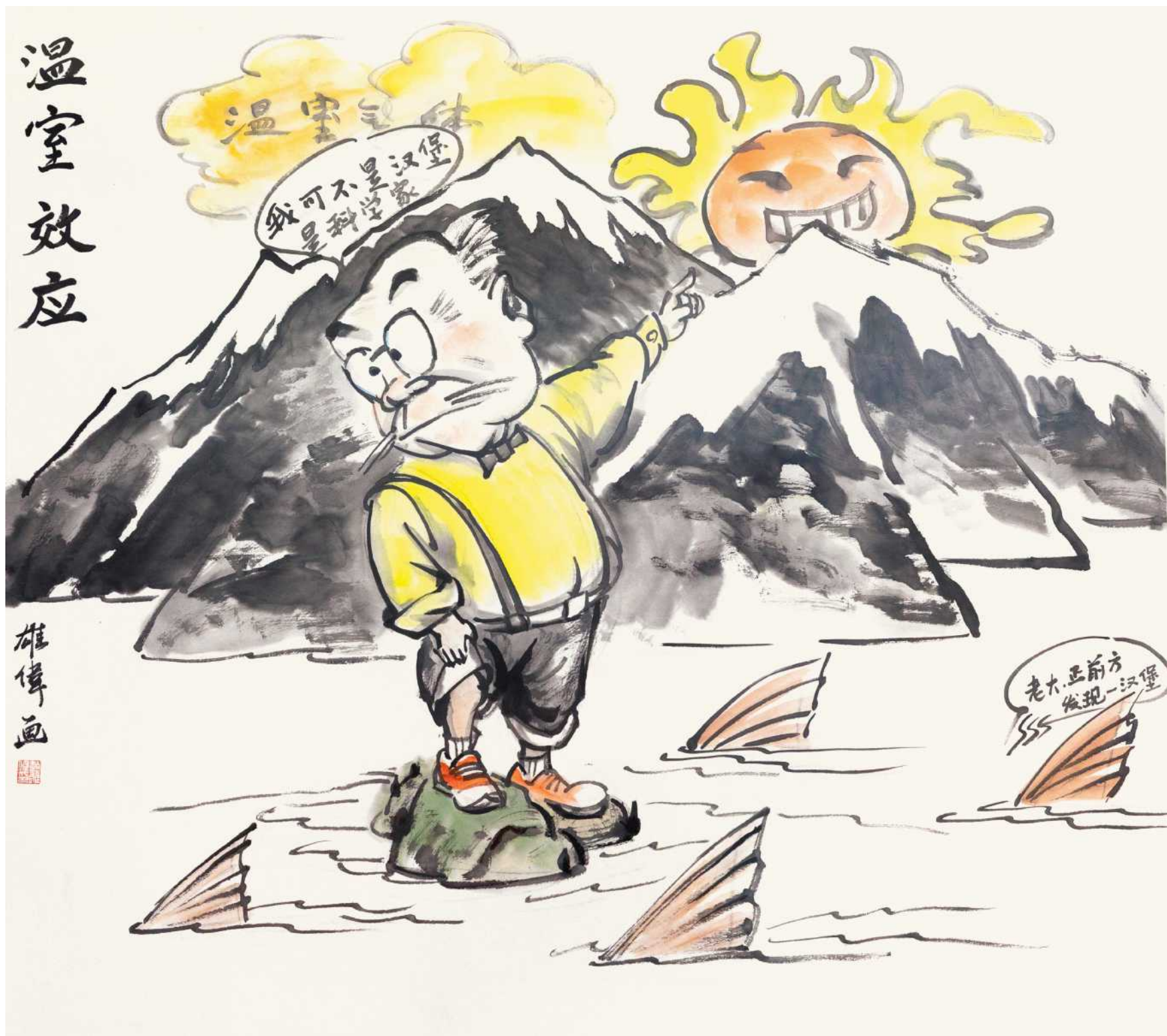
温室效应
